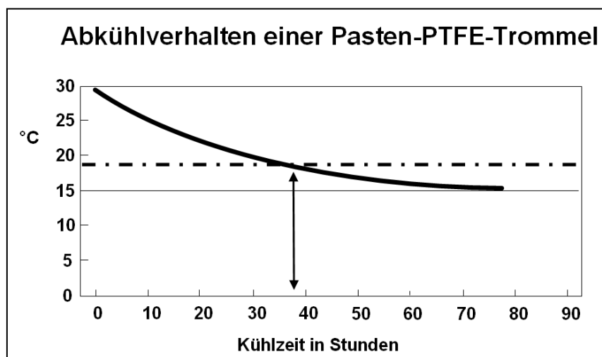
Abb. 7: Abkühlzeit einer 25 kg Pasten-PTFE-Trommel bei einer Lagertemperatur von 15 °C
