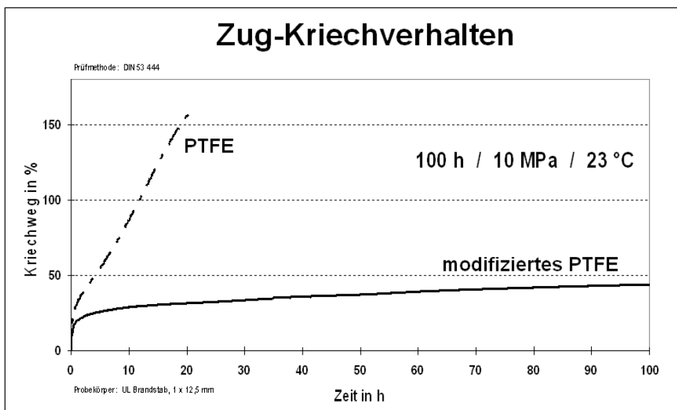
Abb. 2: Reduziertes Zug-Kriechverhalten von modifiziertem PTFE
